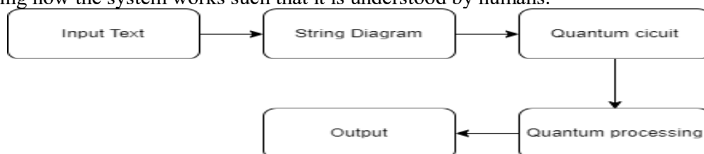
Fig. (QNLP)
